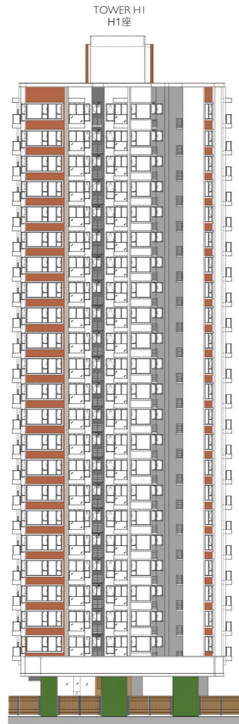
ELEVATION D - TOWER H1 立面圖 D - H1座
