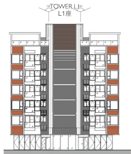
ELEVATION G - TOWER L1 立面圖 G - L1座
